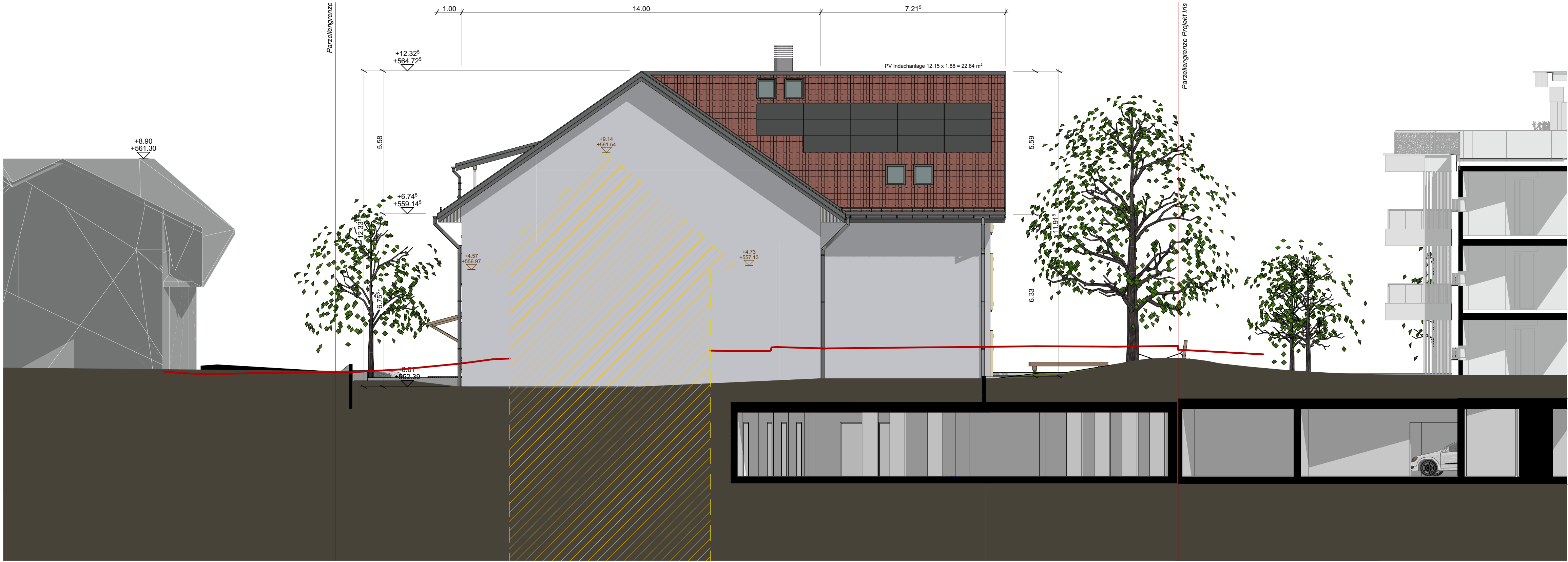
A-03 Ostansicht (Brandmauer) 1:100
