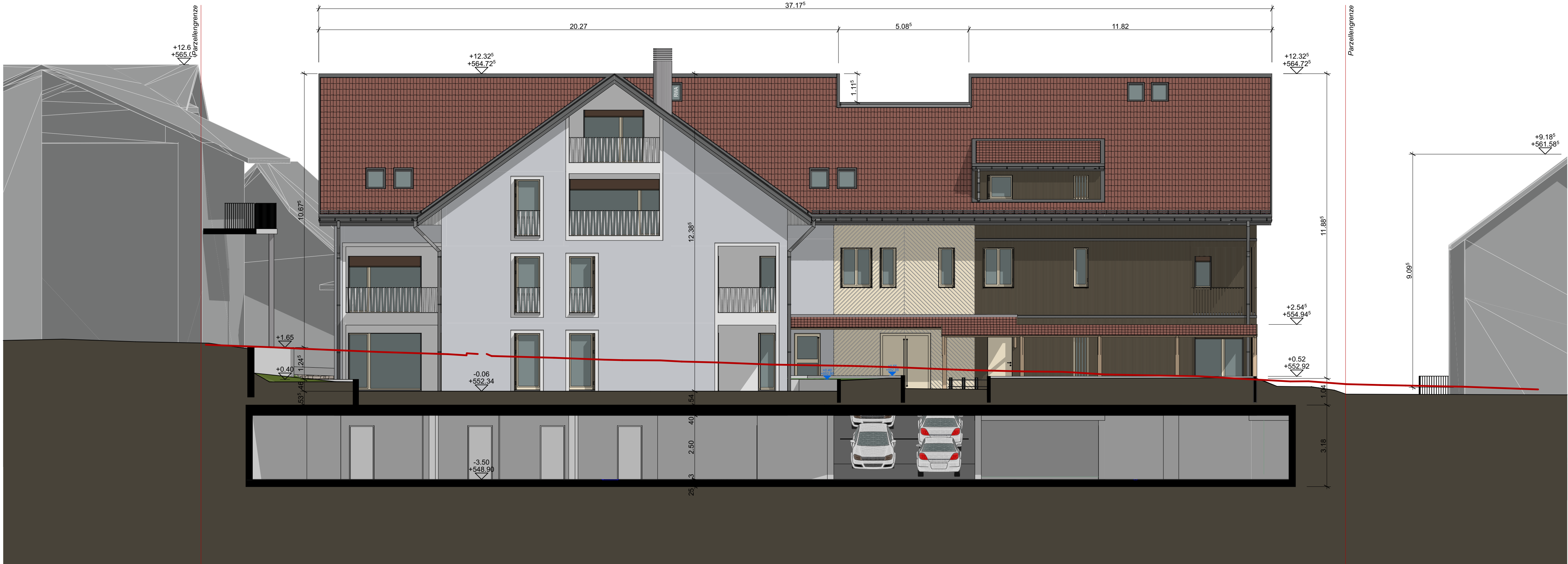
A-04 Nordansicht 1:100
