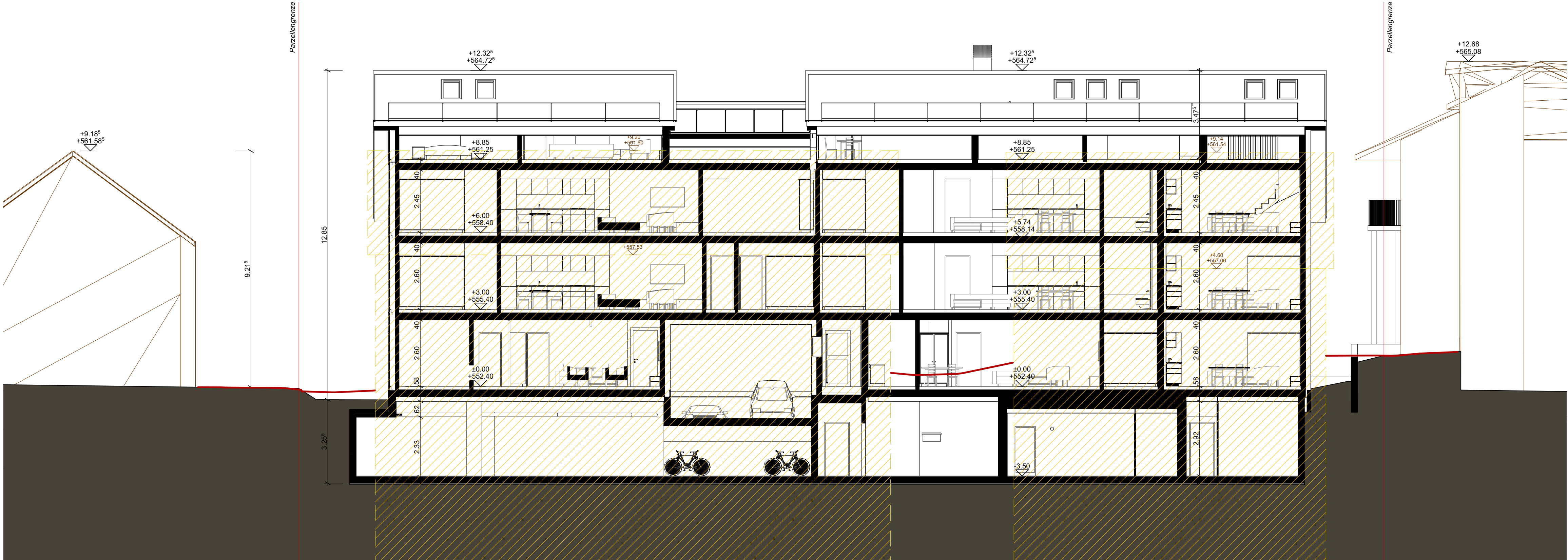
E - E Längsschnitt I 1:100
