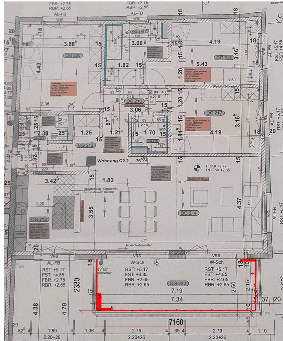
Grundriss Whg 1. OG Mst.: 1:100
