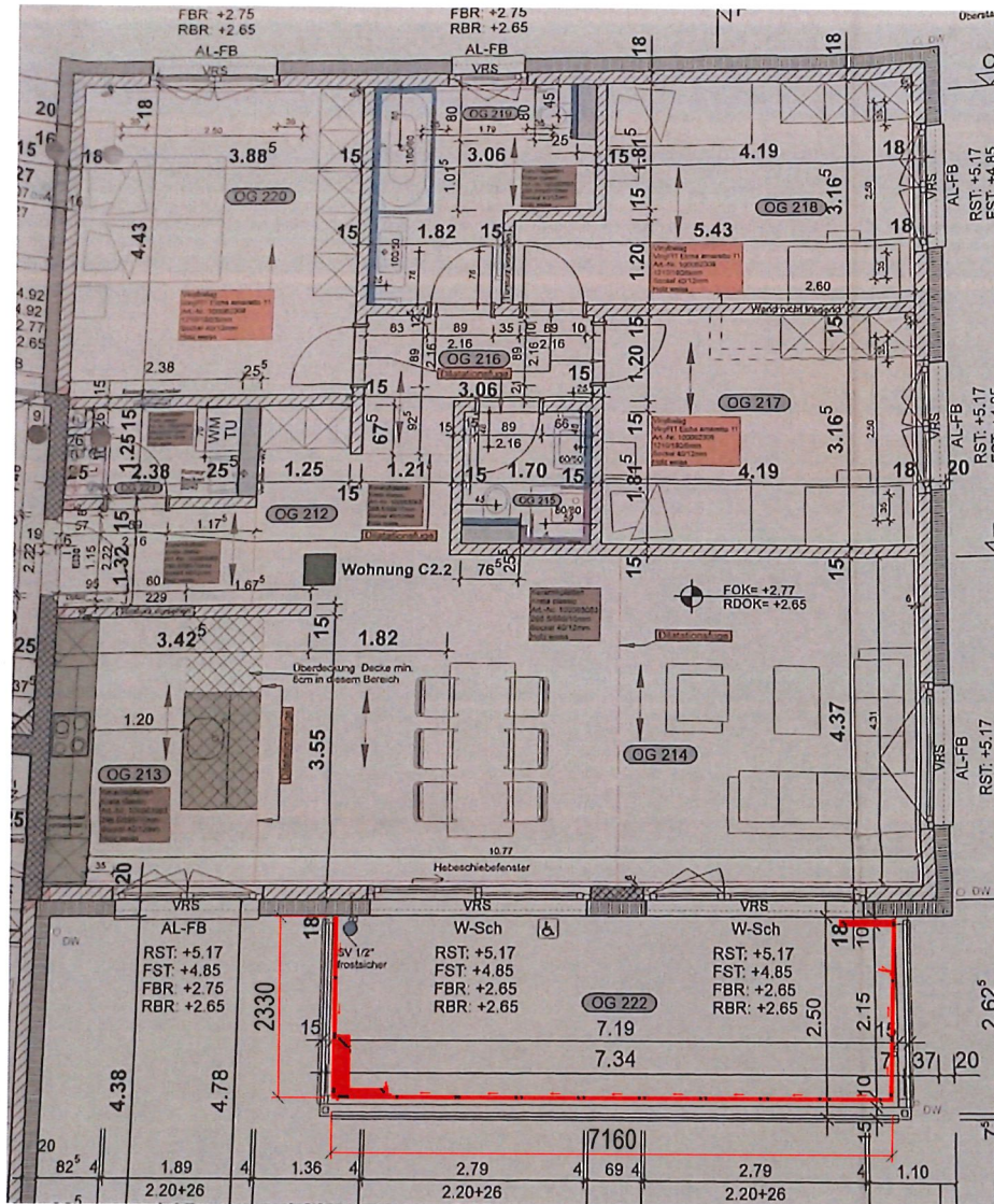
Grundriss Whg 1. OG Mst.: 1:100
