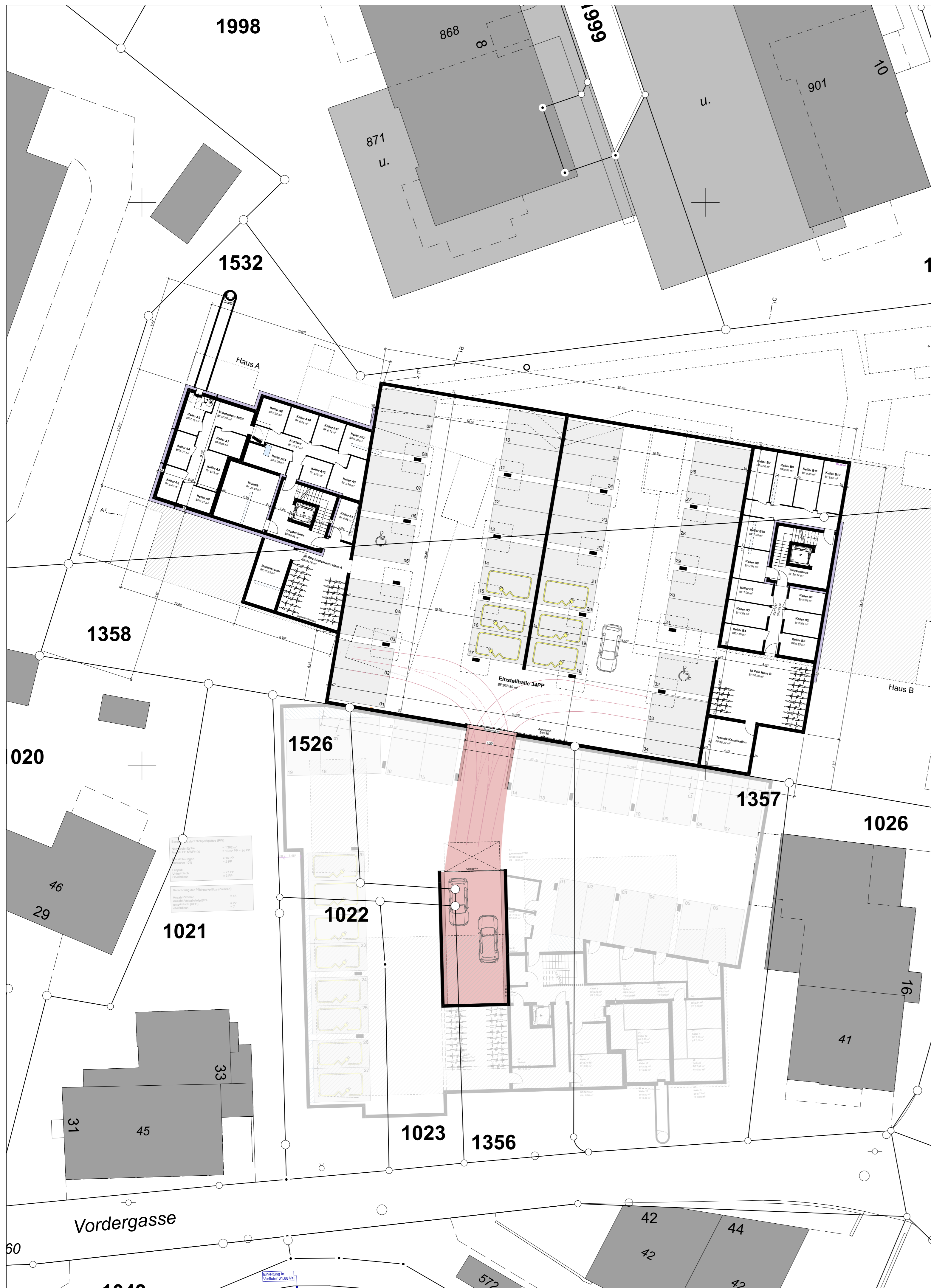
-1. Erschliessung durch Projekt Vordergasse 1:200
