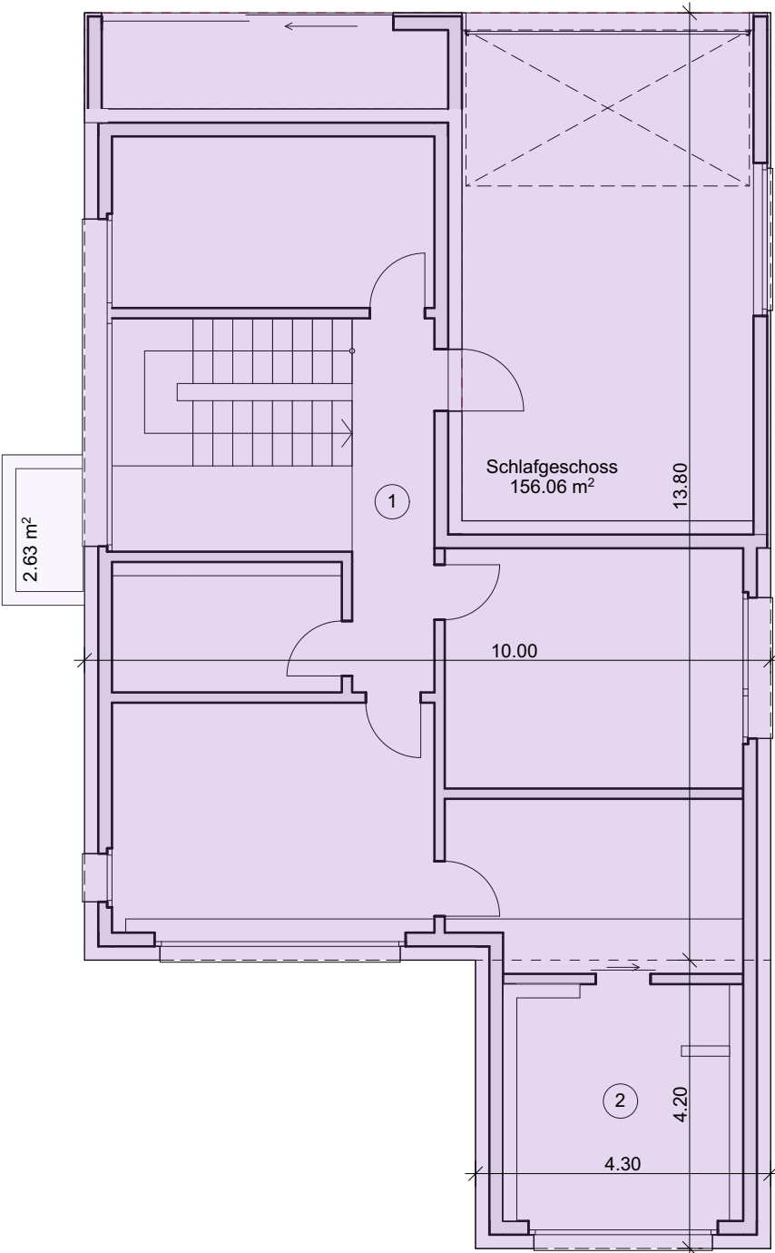
SCHEMA GEBÄUDEVOLUMEN SCHLAFGESCHOSS MST 1:100
