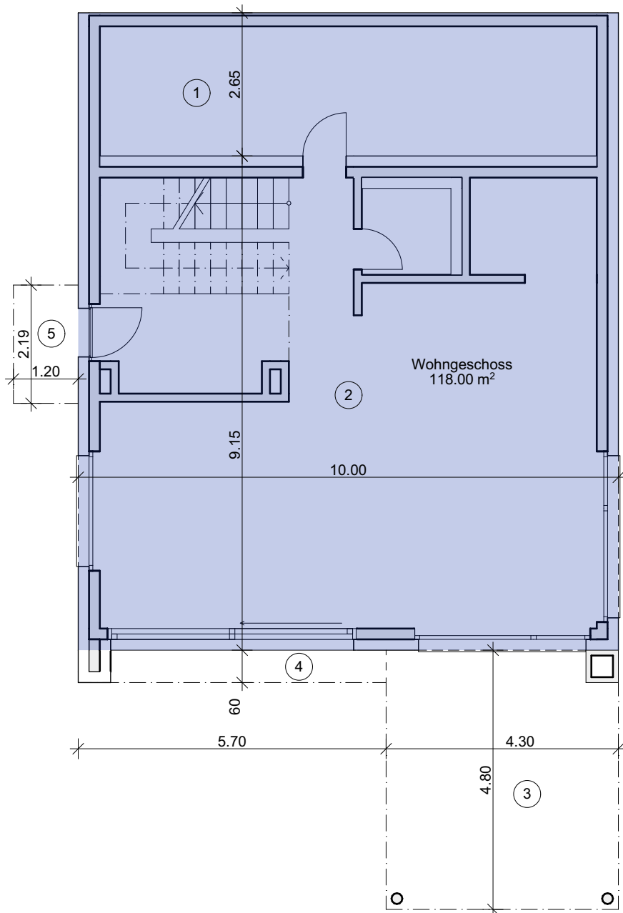
SCHEMA GEBÄUDEVOLUMEN WOHNGESCHOSS MST 1:100
